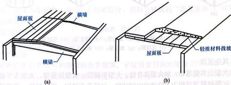
图 11-6 屋面坡度的形成
