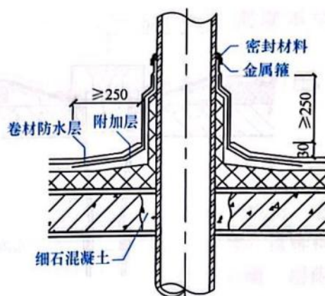
图 11-16 伸出屋面管道
