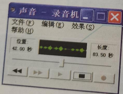
图 1-6-4 正在录音
