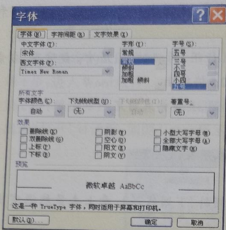
图 1-2-5 “字体”对话框
