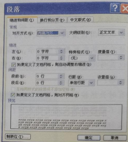
图 1-2-6 “段落”对话框
