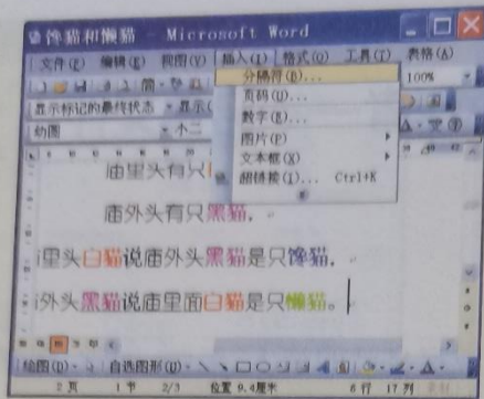
图 1-3-1 插入分隔符
