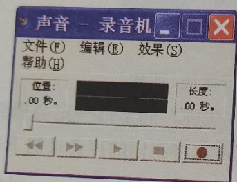
图 1-6-3 “录音机”窗口
