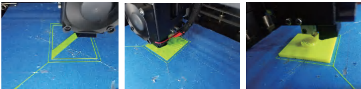
图3-13 三维打印机优先打印底座，再构建圆柱
