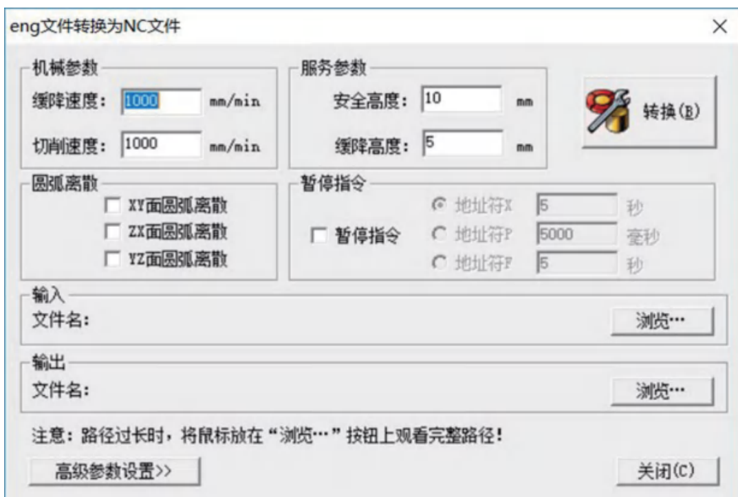
图3-45 将刀具路径转化为机器可识读的格式
