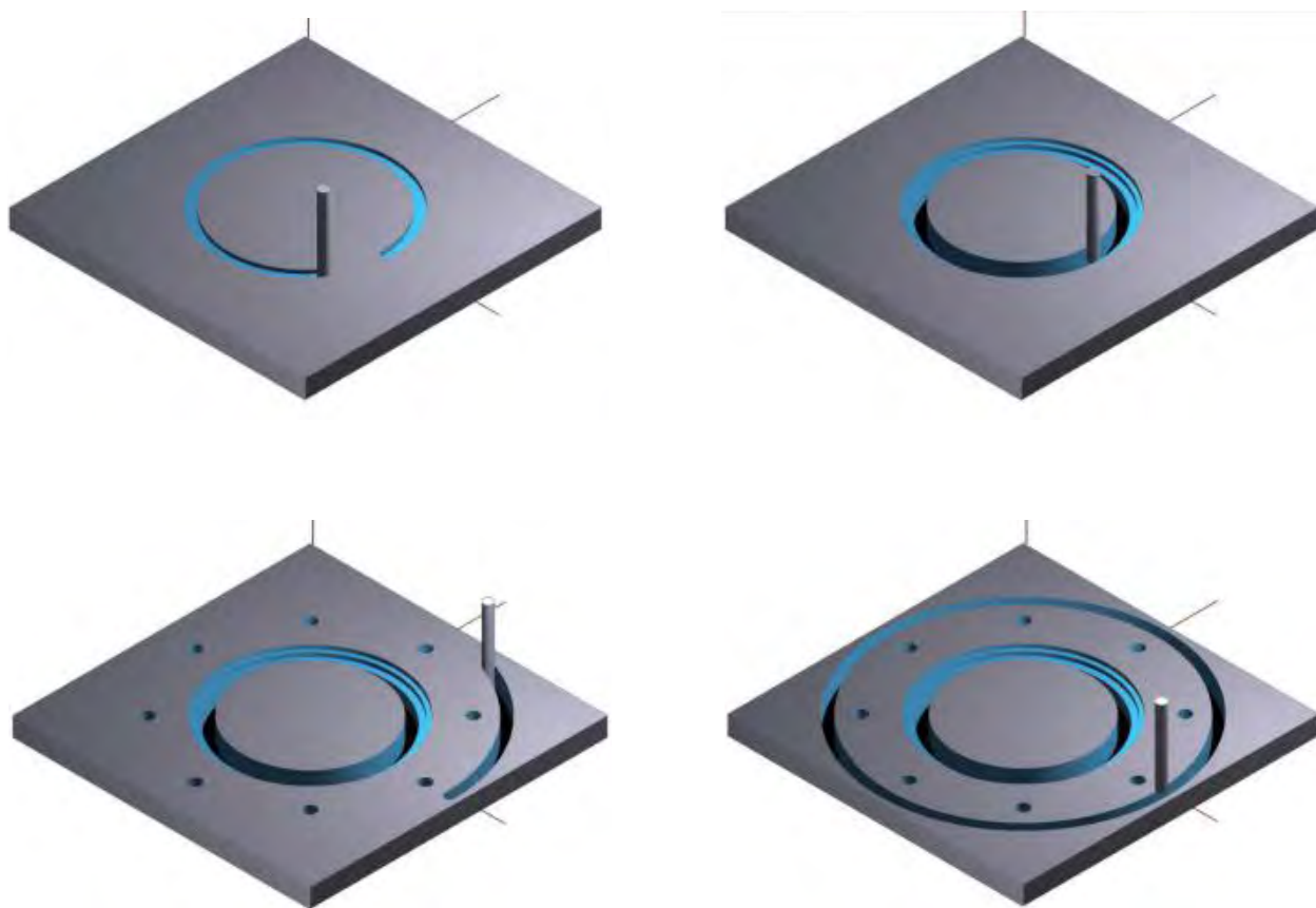
图3-44 模拟仿真加工，检验工作路径
