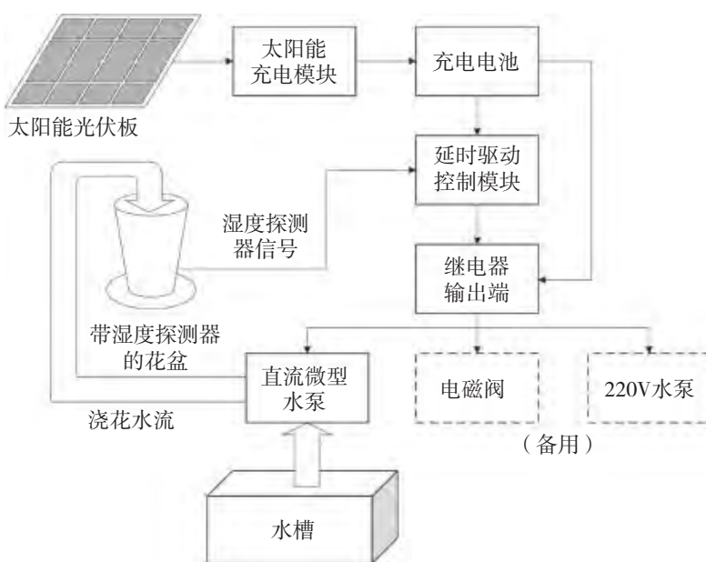
图1-8 作品的工作原理
