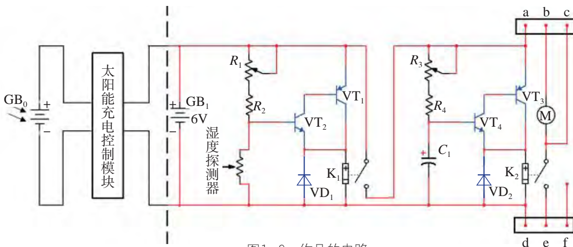
图1-9 作品的电路
