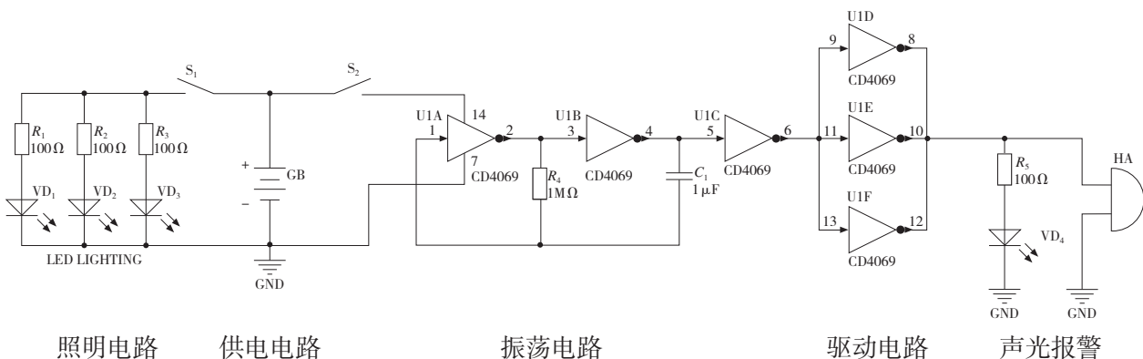
图3-49 方案2的电路图
