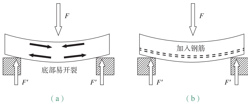
图 1-31 钢筋混凝土梁示意图
