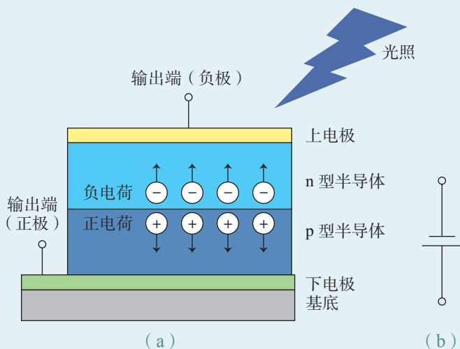
图2-22 太阳能电池结构和等效电路示意图
