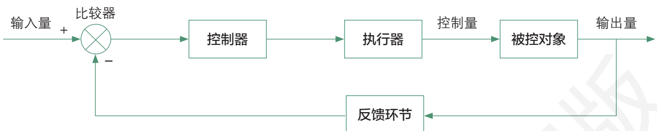
图4-16 闭环控制系统
