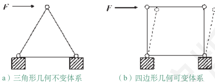
图1-25 结构的形状与稳定性
