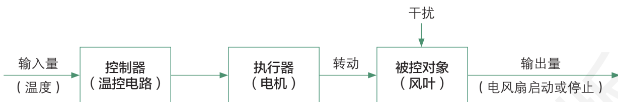
图4-22 温控电风扇控制系统框图
