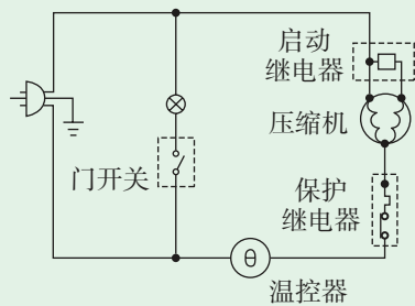
图3-4 电冰箱电气系统示意图
