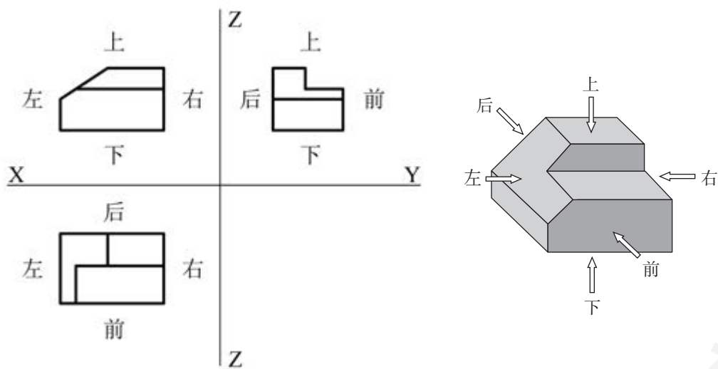
图2-48 平面图中的空间方位体现
