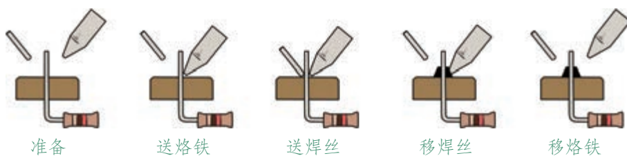
图3-50 五工序法
