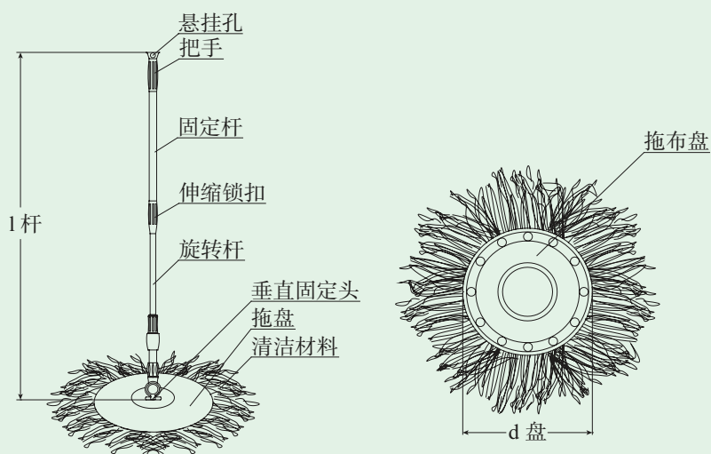
拖把结构示意图
