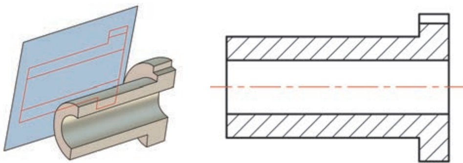
图2-61 剖视图
