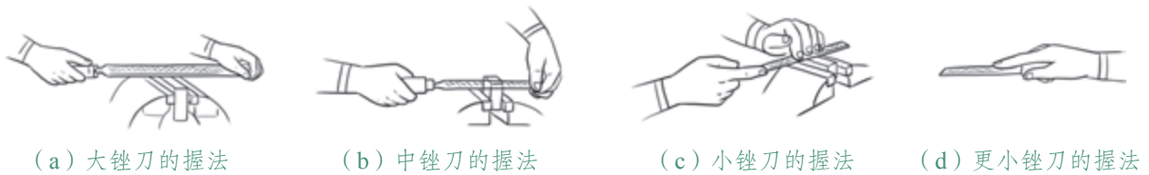
图3-31 锉刀的握法
