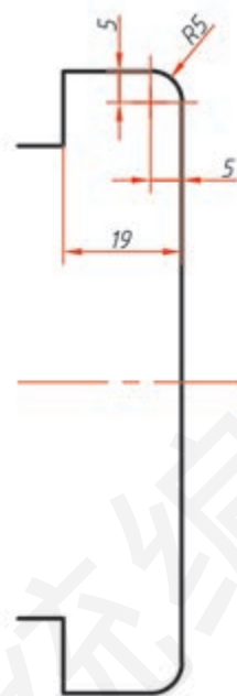
图2-73 循迹小车底板左右上侧圆角
