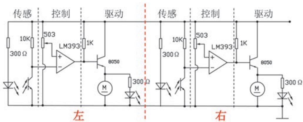
图2-35 循迹小车电路原理图
