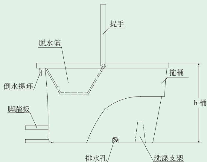
拖桶结构示意图
