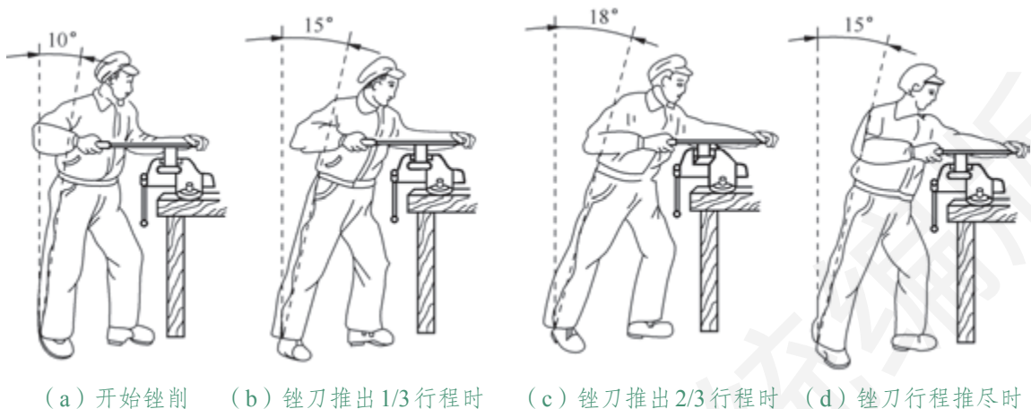
图3-32 锉削过程身体的姿势
