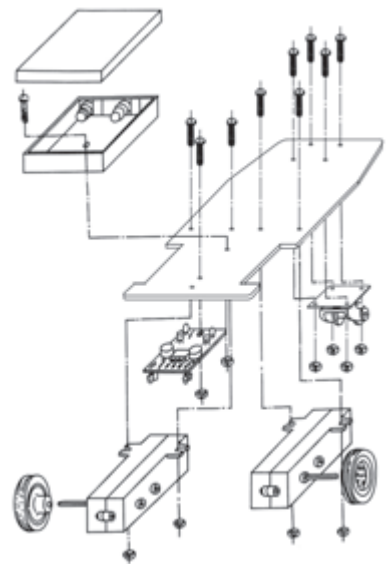
图3-57 循迹小车装配示意图
