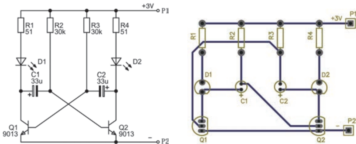
图3-51 简易双闪灯电路
