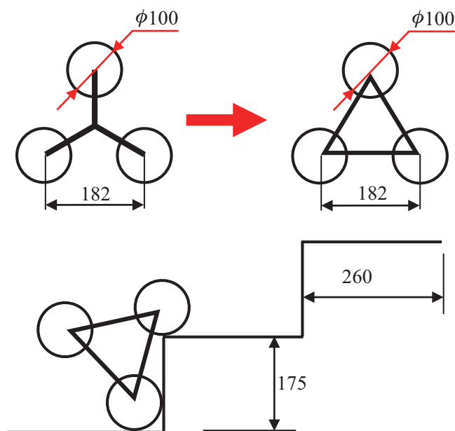
图2-29 完善构思方案
