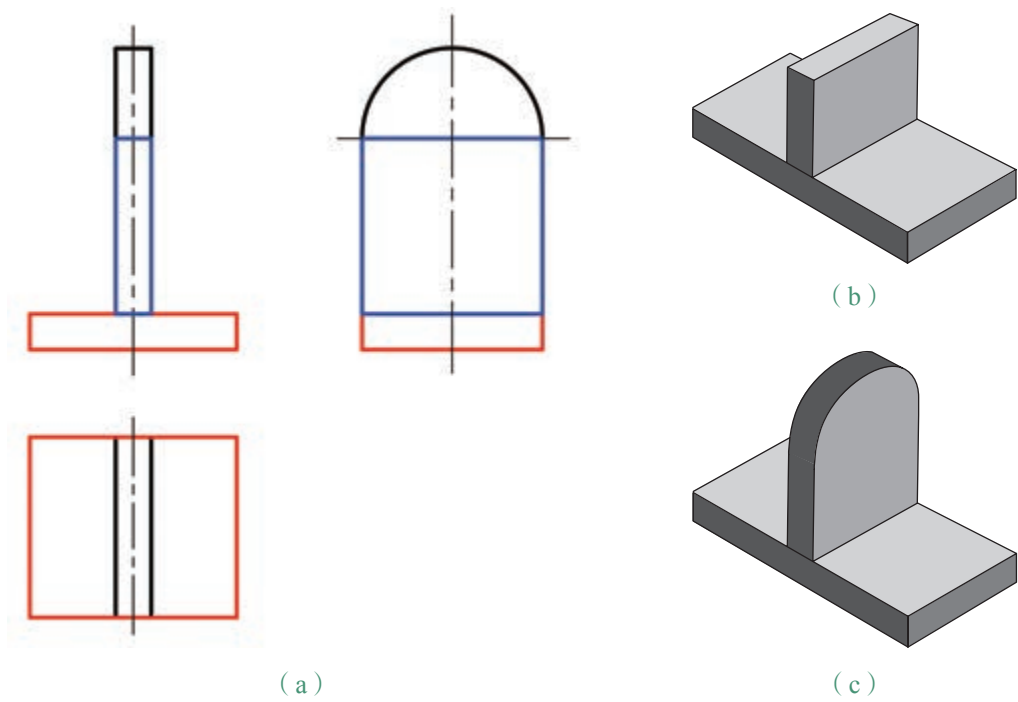
图2-58 识读三视图
