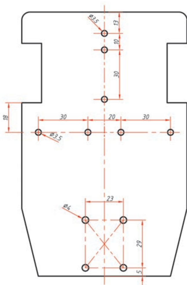
图2-75 循迹小车底板圆孔绘制图
