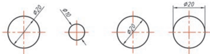
图2-66 直径标注
