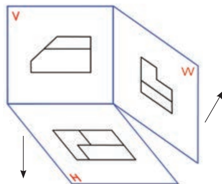
图2-47 三视图的平面展开
