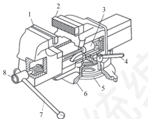
1 活动钳口 2 固定钳口 3 螺母 4 锁紧手柄 5 锁紧盘 6 转盘座 7 拔杆 8 丝杠
