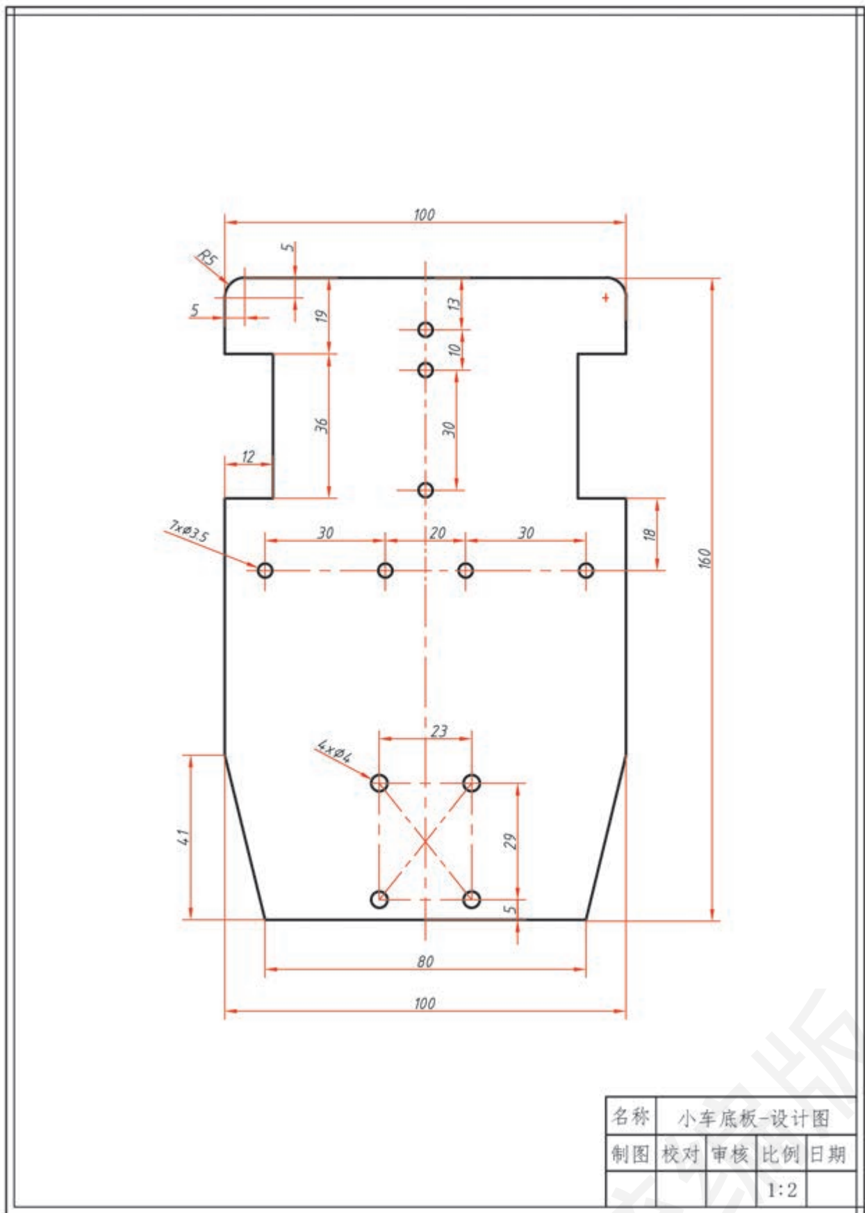
图2-77 循迹小车底板设计图
