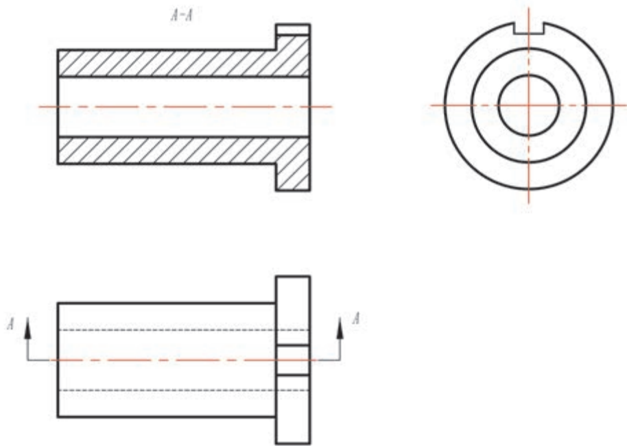
图2-62 零件剖视图
