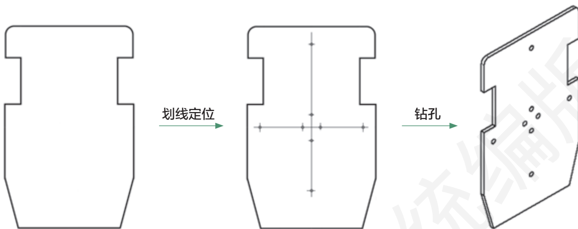
图3-40 循迹小车底板的钻孔操作
