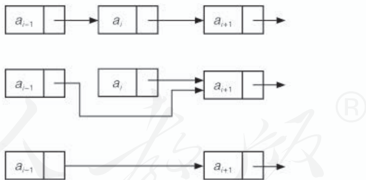
图2.2.13 删除节点的指针变化示意图
