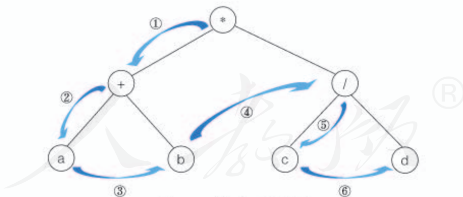
图 3.5.14 先根序遍历示意图
