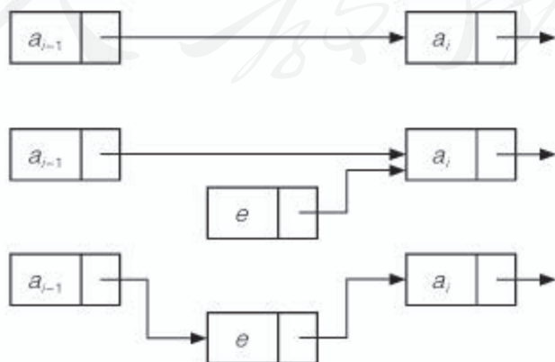
图 2.2.12 在单链表中插入节点的指针变化示意图
