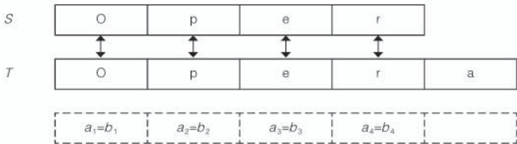
图 3.4.5 字符串比较 (2)
