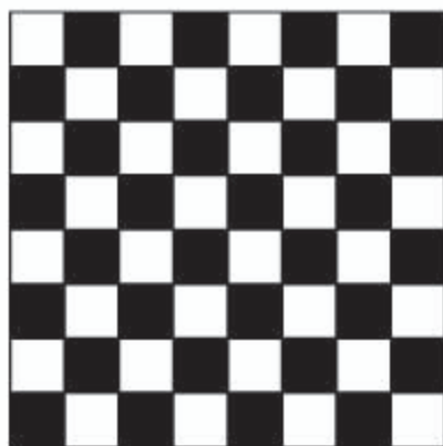
图 1.1.3 棋盘示意图
