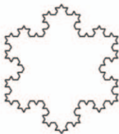
图4.3.7 雪花曲线
