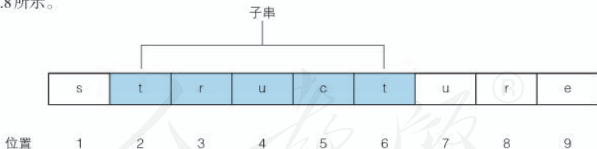
图3.4.8 获取子串
