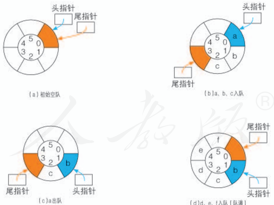
图3.3.11 循环队列示意图
