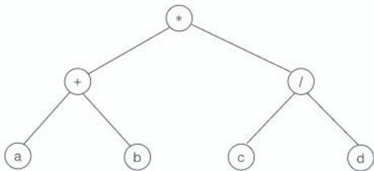
图 3.5.13 表达式二叉树
