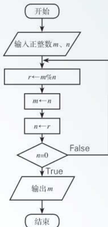
图 4.2.6 求最大公因数的算法流程图
