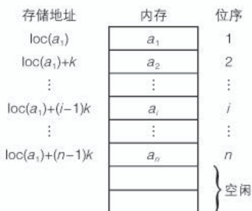
图2.2.3 顺序存储结构示意图
