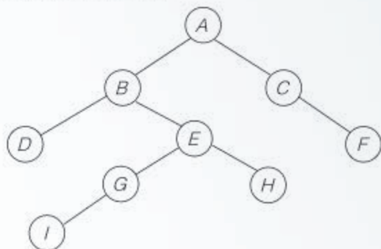
图 3.5.11 二叉树结构
