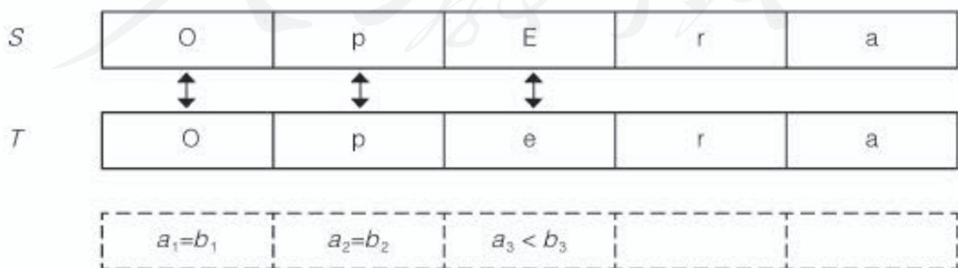
图 3.4.6 字符串比较 (3)
