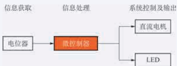
图 2.35 调速小风扇系统框图
