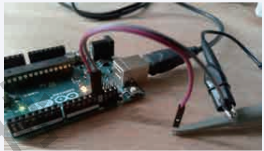
图 1.36 示波器接法
