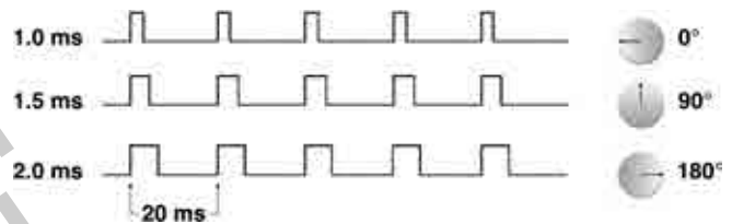
图 2.34 舵机的旋转角度控制
