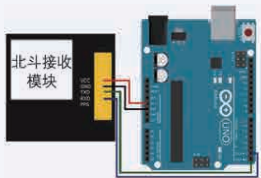
图 3.5 Arduino Uno与北斗接收模块连接图
