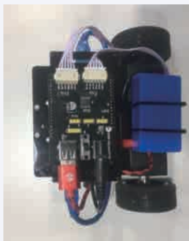
图 4.5 运动小车的完整组装
