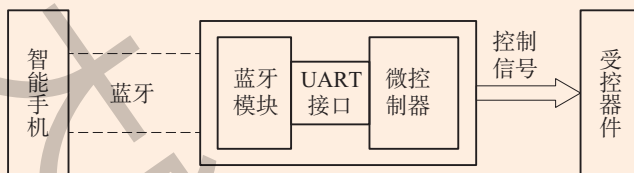
图 3.16 智能手机控制示意图
