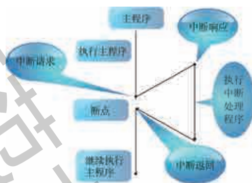
图 2.4 中断流程示意图
