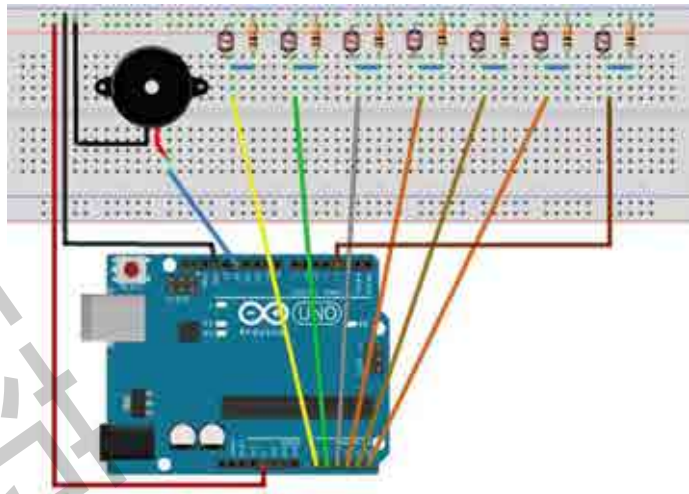
图 2.27 光敏电子琴
