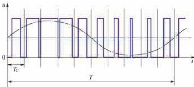
图 2.28 PWM 示意图
