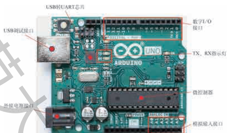
图 1.17 Arduino Uno 开发板的组成
