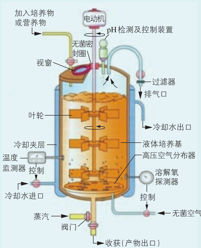
A. 工业发酵罐的结构与控制装置示意图
