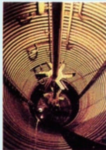
工业发酵罐内部的叶轮及加热或冷却的管道
