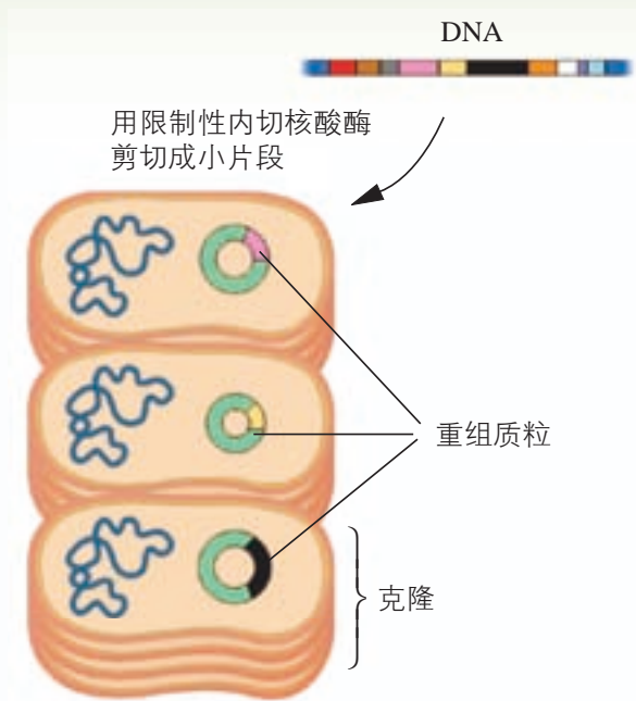
图4-10 构建基因组文库示意图
