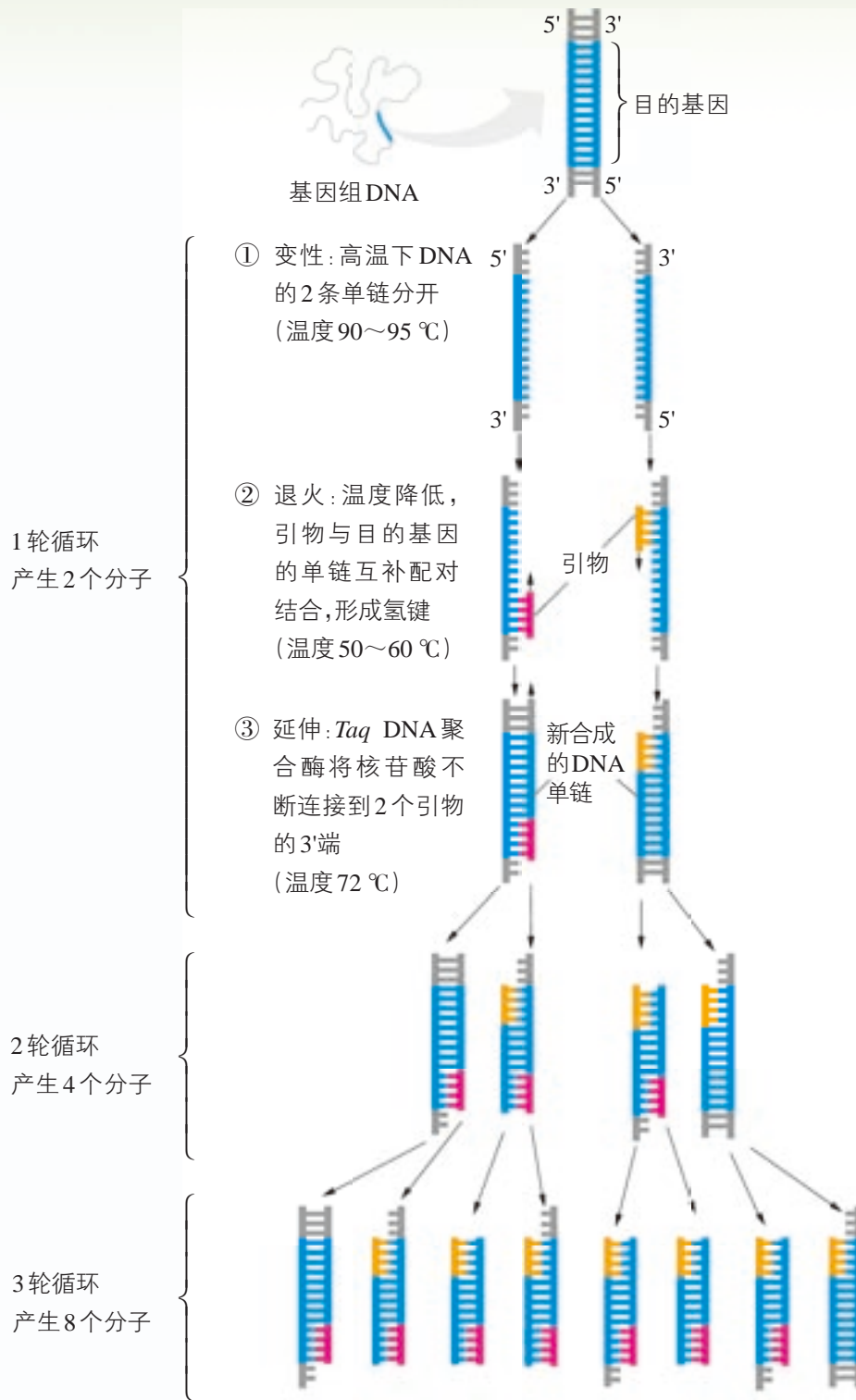
图4-11 PCR原理示意图
