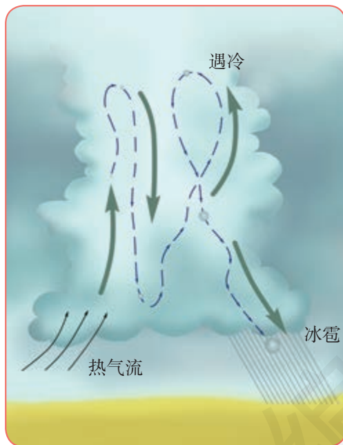
冰雹形成过程示意图
