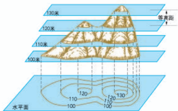
图1.36 等高线示意
