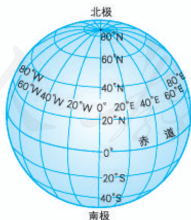
图1.12 经纬网
