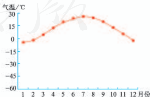
图3.12 气温年变化
