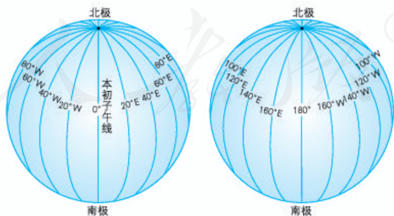
图1.9 经线和经度
