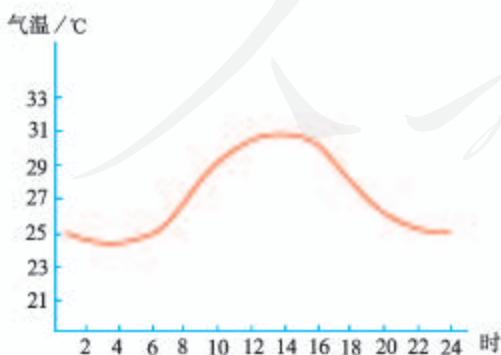
图3.11 气温日变化
