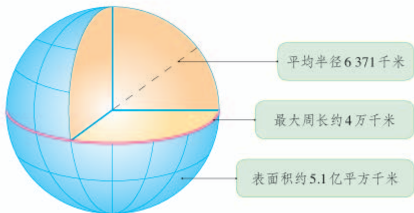
图1.2 地球的大小
