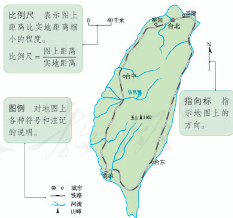
图1.22 台湾岛地图
