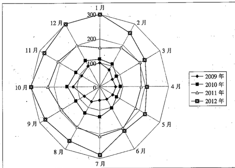
图中三个圆的半径分别为 100、200 和 300 万元
